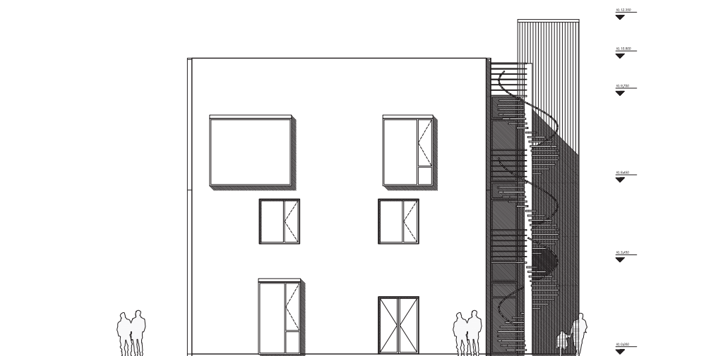
FACADE MOD NORD
